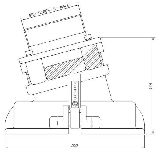
Dimensions / Dimensiones
