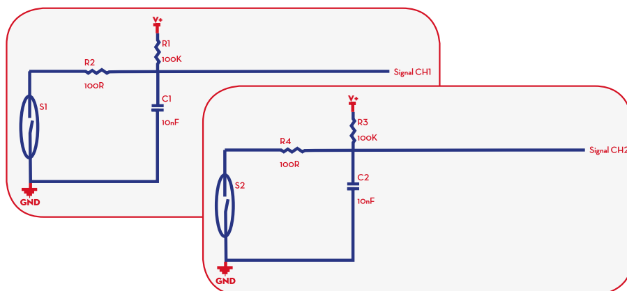
ESQUEMA ELÉCTRICO
